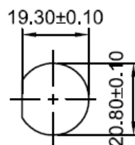
Empfohlene Aussparung für USB Recommended cut-out for USB
