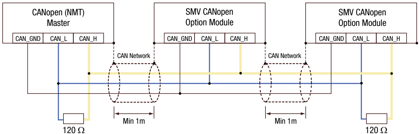
Abbildung 6: Netzwerk Schaltplan
