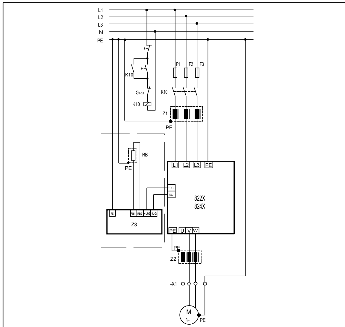
FIG 4-6 Leistungsanschlüsse 822X/824X
