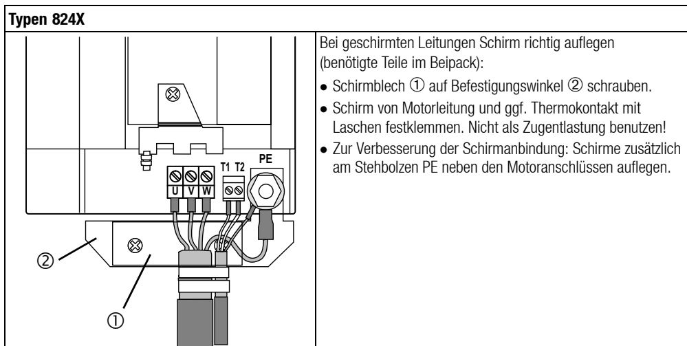
FIG 4-5 Vorschlag für Motoranschluß bei 824X
