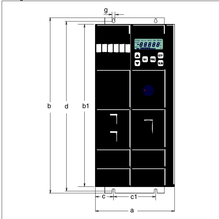
Abmessungen der Geräte 8201G bis 8202G in mm
